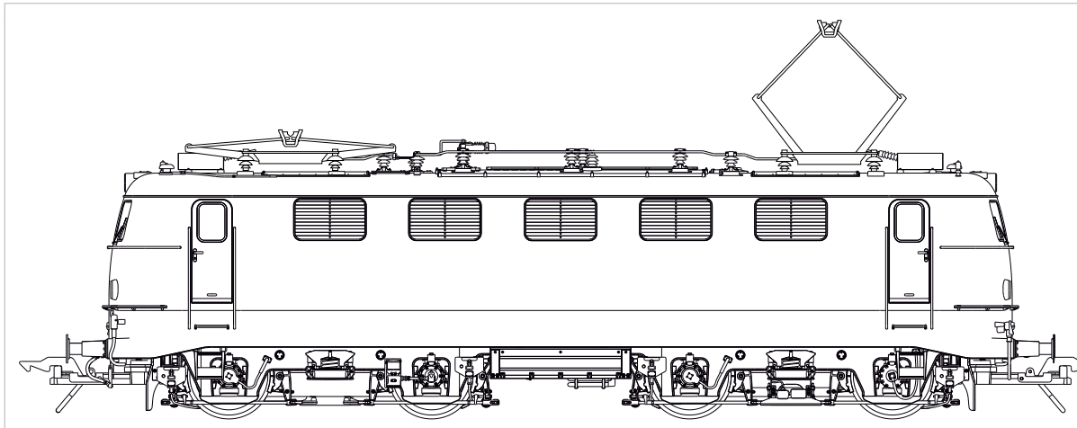
Art.Nr. 40300-01 - Elektrolokomotive E 41 - Konstruktionszeichnung
